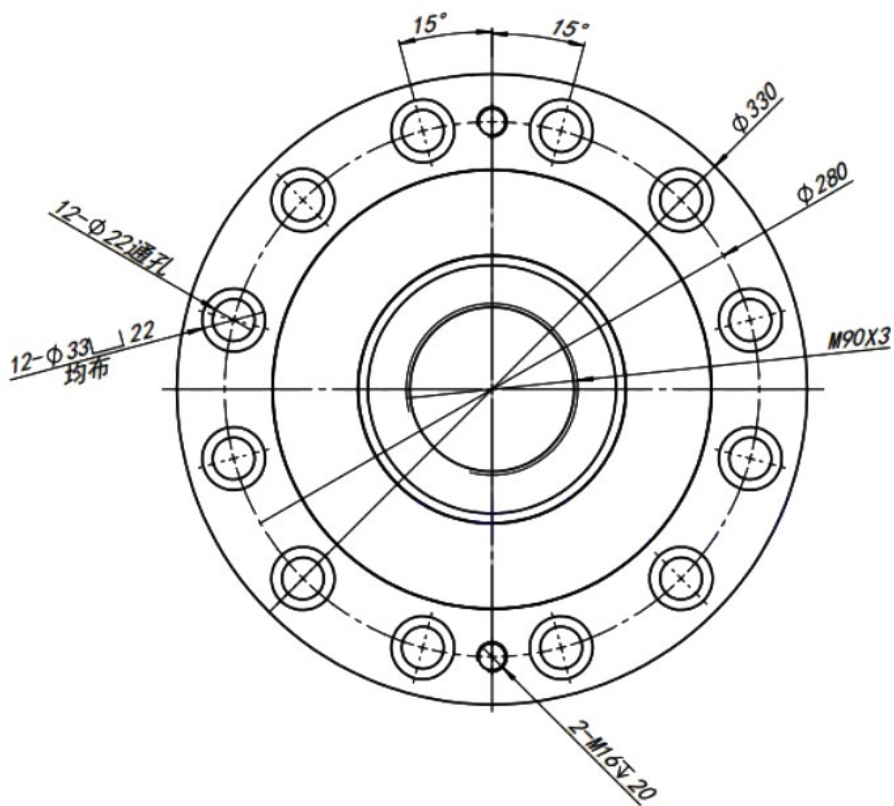
100t外形尺寸
