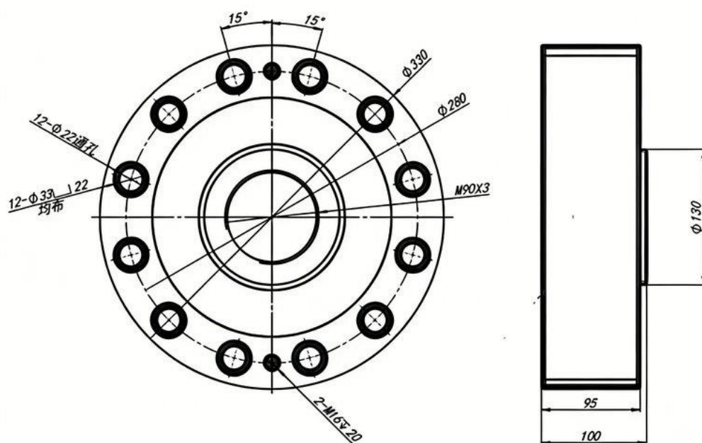
100t外形尺寸
